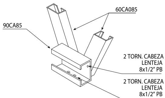
PERSPECTIVA DET.1 S/E
