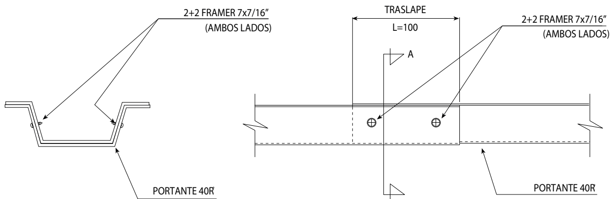
ELEVACIÓN EMPALME PORTANTE 40R
