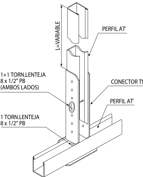
PERSPECTIVA DET.1 S/E
