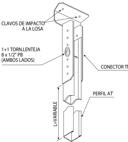
DETALLE CONEXIÓN A LOSAS S/E
